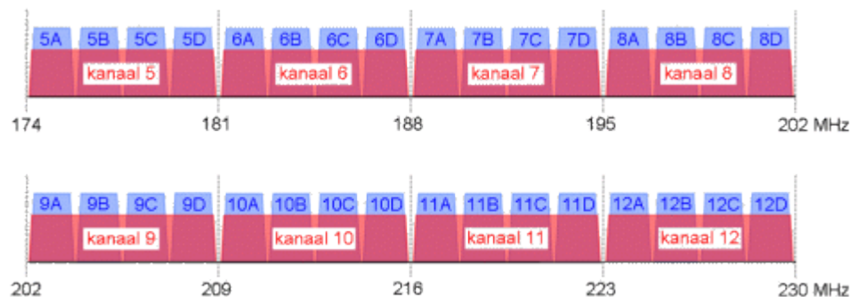
VHF – band III kanaalindeling voor T-DAB+.
